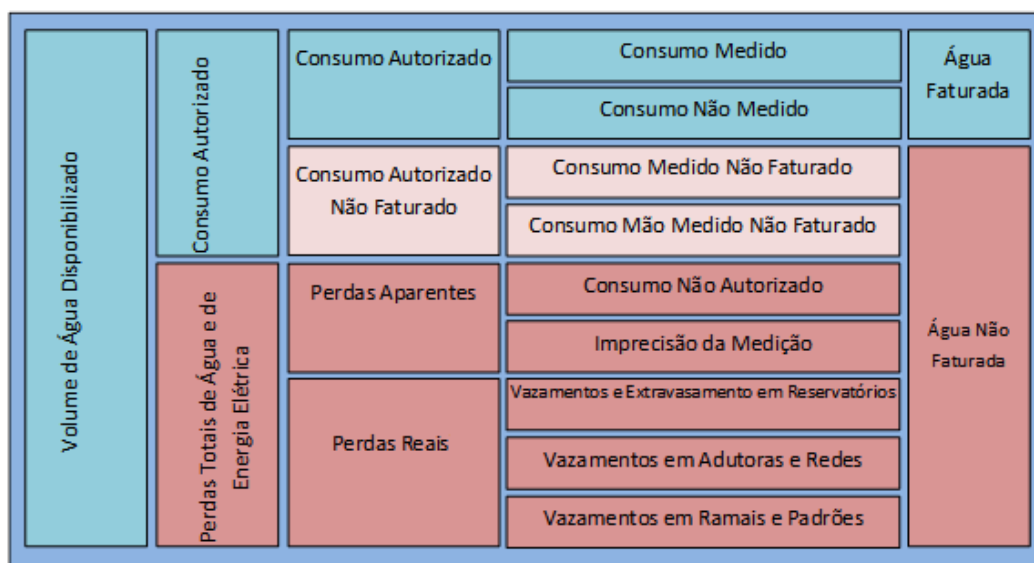
Figura 1: Balanço Hídrico
