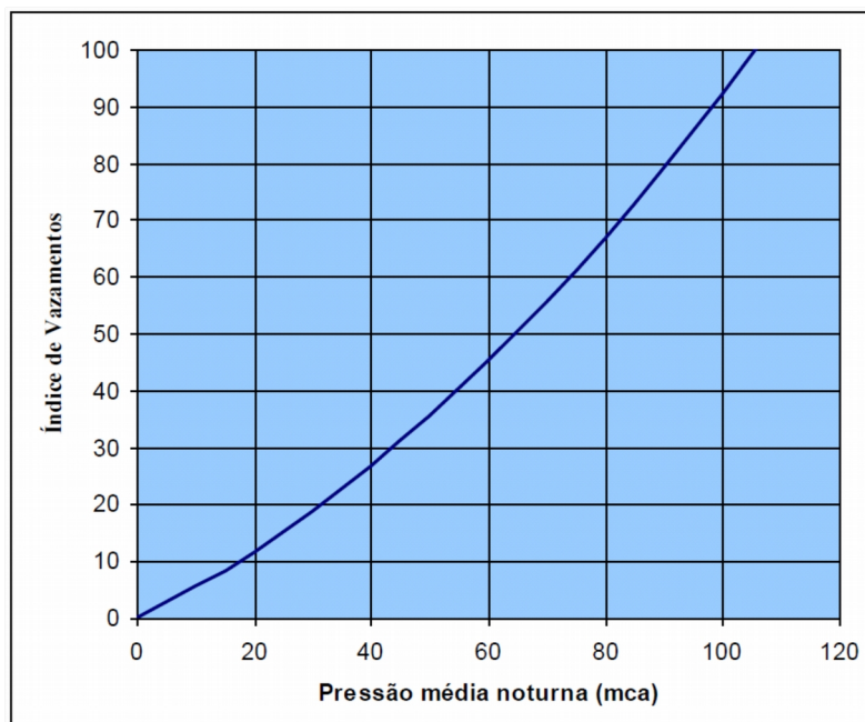
Figura 1: Relação entre pressão e volume perdido
