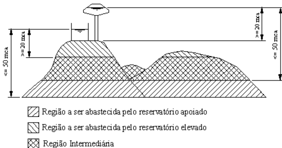
Figura 1: Esquema de Setorização Clássica
