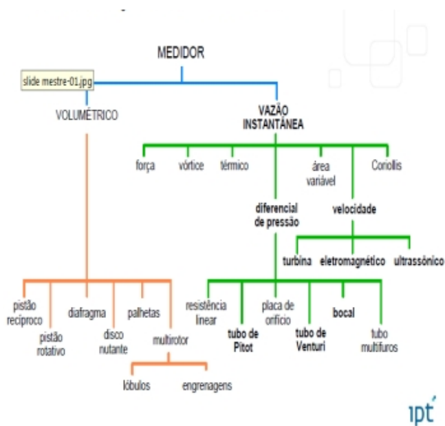
Figura 1: Classificação de Medidores de Vazão
