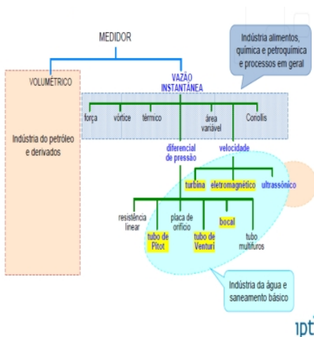
Figura 1: Campo de aplicação de medidores
