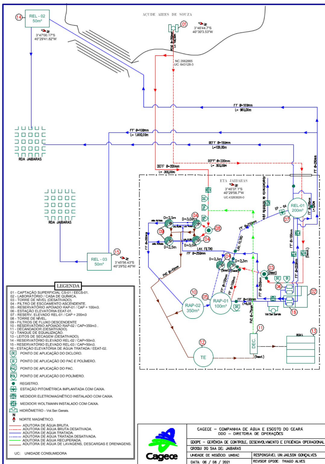
Figura 1 - Croqui do SAA da Localidade de Jaibaras
