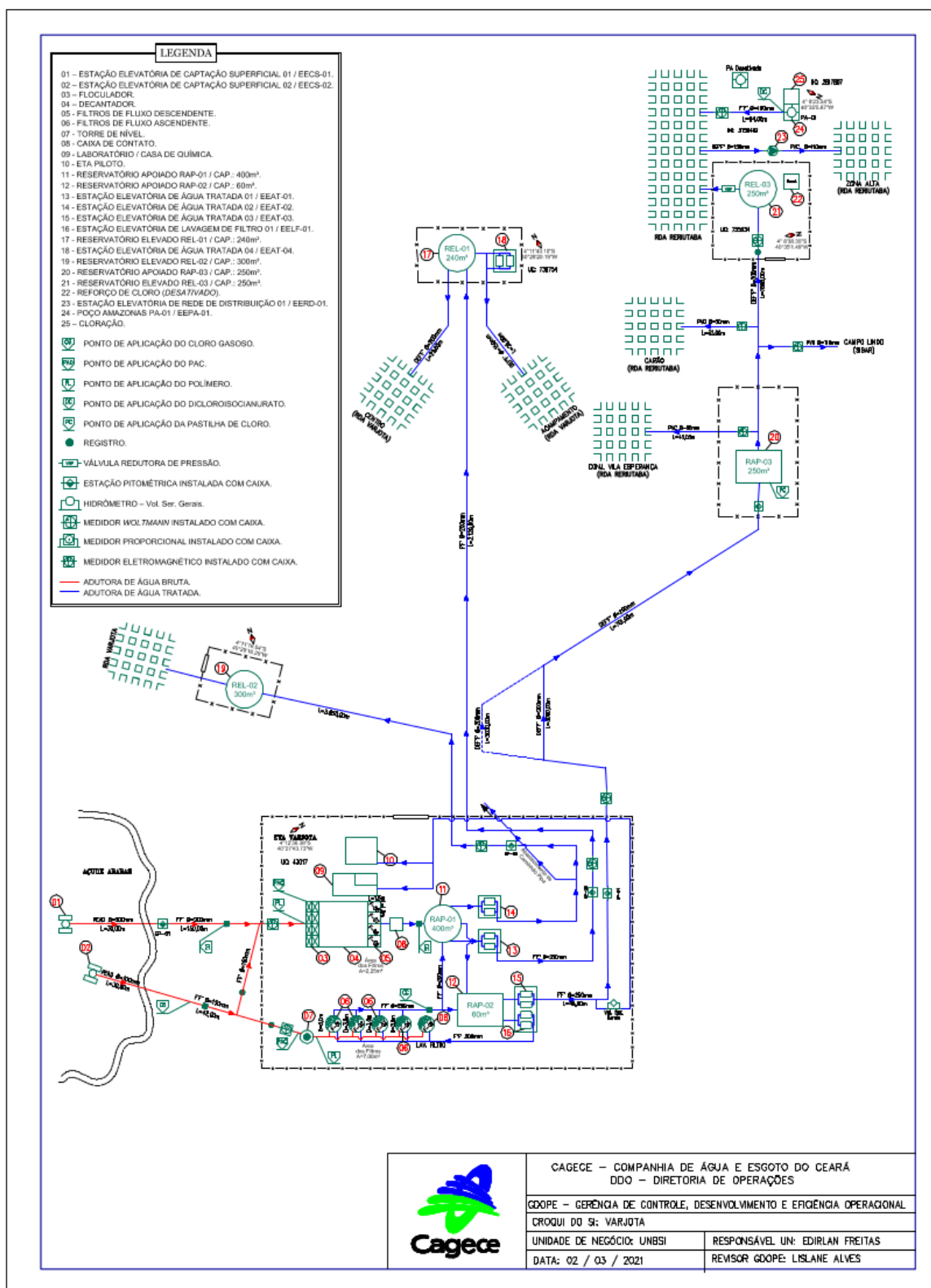
Figura 1 - Croqui do SAA de Varjota
