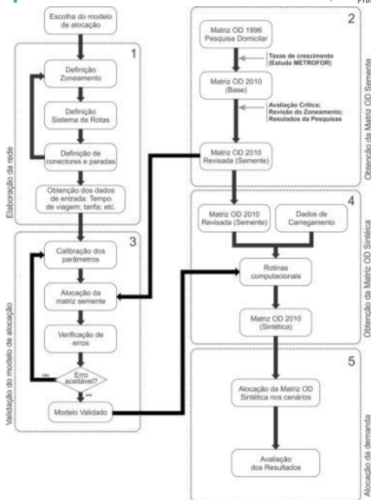
Figura 1.11: Fluxograma das atividades desenvolvidas na modelagem
