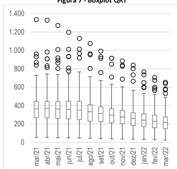
Figura 7 - Boxplot QRT
