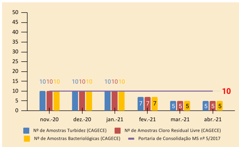
Figura 3 - Avaliação do Monitoramento da Qualidade da água tratada realizado pela CAGECE, na rede de distribuição do SAA de Pires Ferreira (Sede) e Localidades de Marruás dos Rosas, Otavilândia e Santo Izidro, no período de nov/2020 a abr/2021, conforme Portaria de Consolidação MS nº 5/2017, com relação ao número de amostras dos exames bacteriológicos, cloro residual livre e turbidez.
