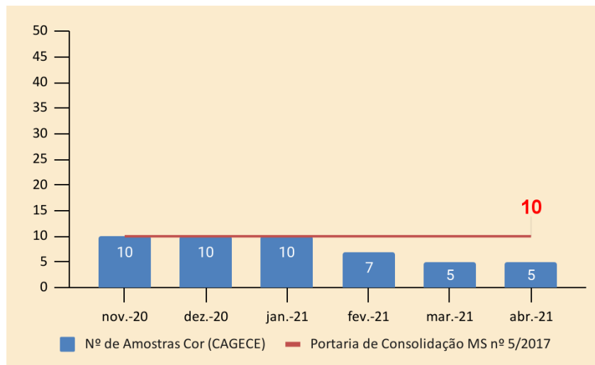
Figura 2 - Avaliação do Monitoramento da Qualidade da água tratada realizado pela CAGECE, na rede de distribuição do SAA de Pires Ferreira (Sede) e Localidades de Marruás dos Rosas, Otavilândia e Santo Izidro , no período de nov/2020 a abr/2021, conforme Portaria de Consolidação MS nº 5/2017, com relação ao número de amostras dos exames cor aparente .
