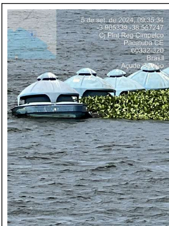
Foto 1 - Captação: Conjuntos motobombas e flutuadores em processo de deterioração.
