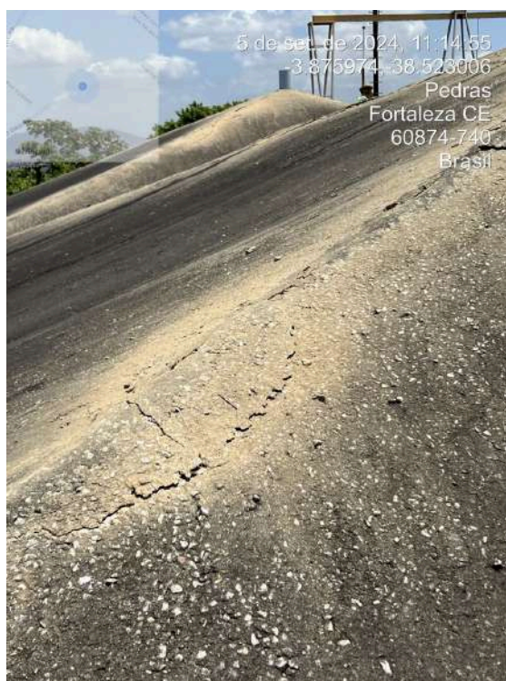
Foto 11 - Reservatório Ancuri: Pontos de corrosão e deterioração do concreto na cobertura dos reservatórios.
