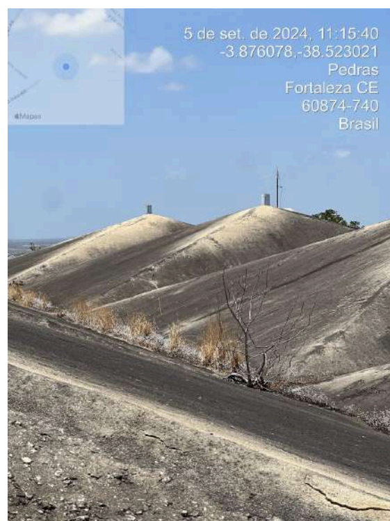
Foto 10 - Reservatório Ancuri: Pontos de corrosão e deterioração do concreto na cobertura dos reservatórios.
