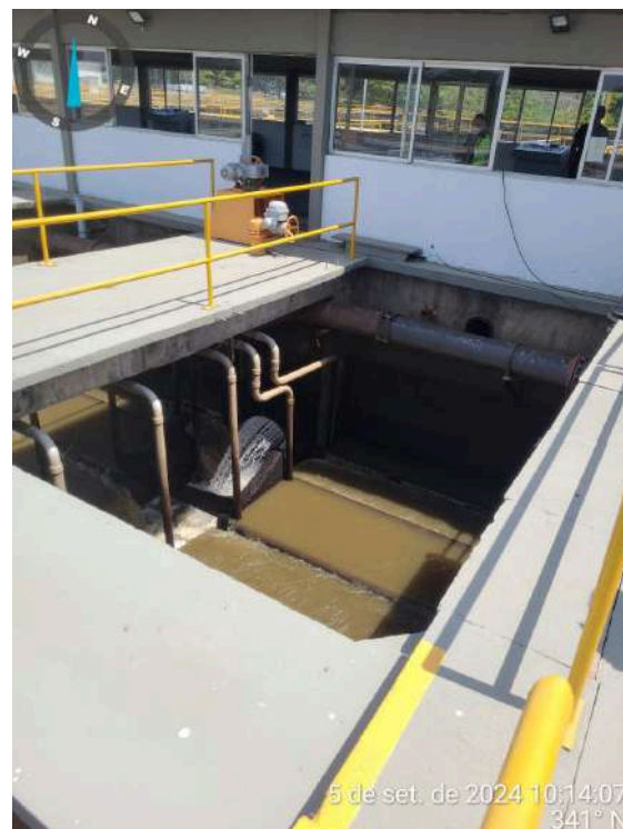
Foto 4 - Filtros: Filtros 1 e 2 com válvulas de registro sem fechar completamente, acarretando perda de água com produtos químicos já adicionados, nos momentos das lavagens.
