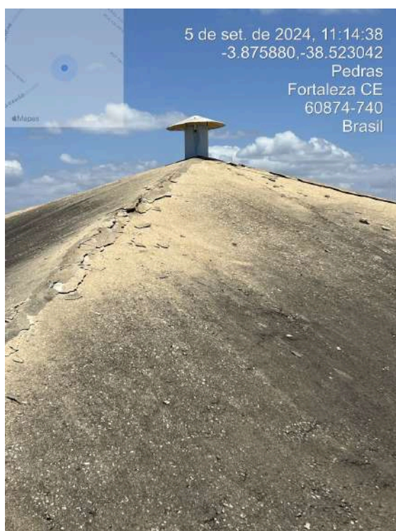
Foto 9 - Reservatório Ancuri: Pontos de corrosão e deterioração do concreto na cobertura dos reservatórios.
