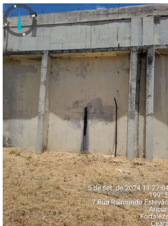
Foto 12 - Reservatório Ancuri: Vazamento nas paredes do reservatório.
