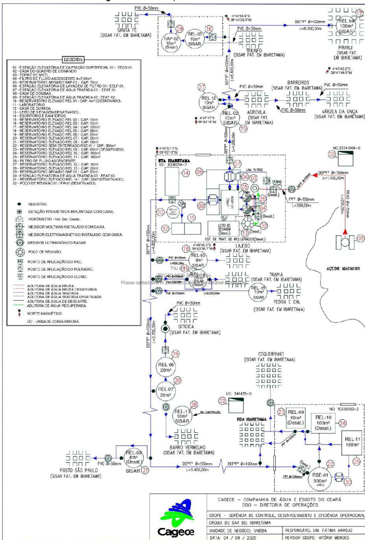
Figura 1 - Croqui do SAA de Ibaretama.
