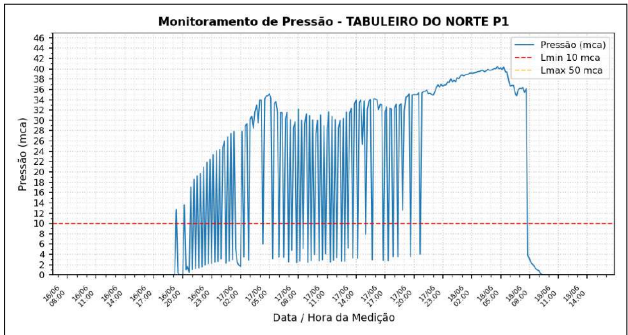
Figura 3 - Monitoramento da pressão no SAA de Tabuleiro do Norte de 16/06/2026 a 18/06/2026, no endereço: Cj Popular Quadra Tres, 75 - A, Joaquim Fernandes Colares.
