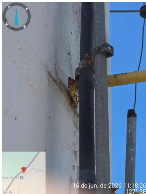
Foto 38 - REL-04: barra sem fixação adequada.
