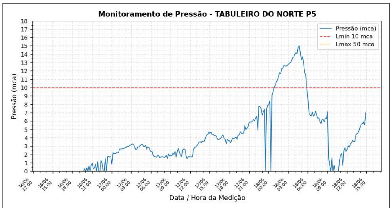
Figura 4 - Monitoramento da pressão no SAA de Tabuleiro do Norte de 16/06/2026 a 18/06/2026, no endereço: Rua Antônio Torquato, 926, Bom Futuro.
