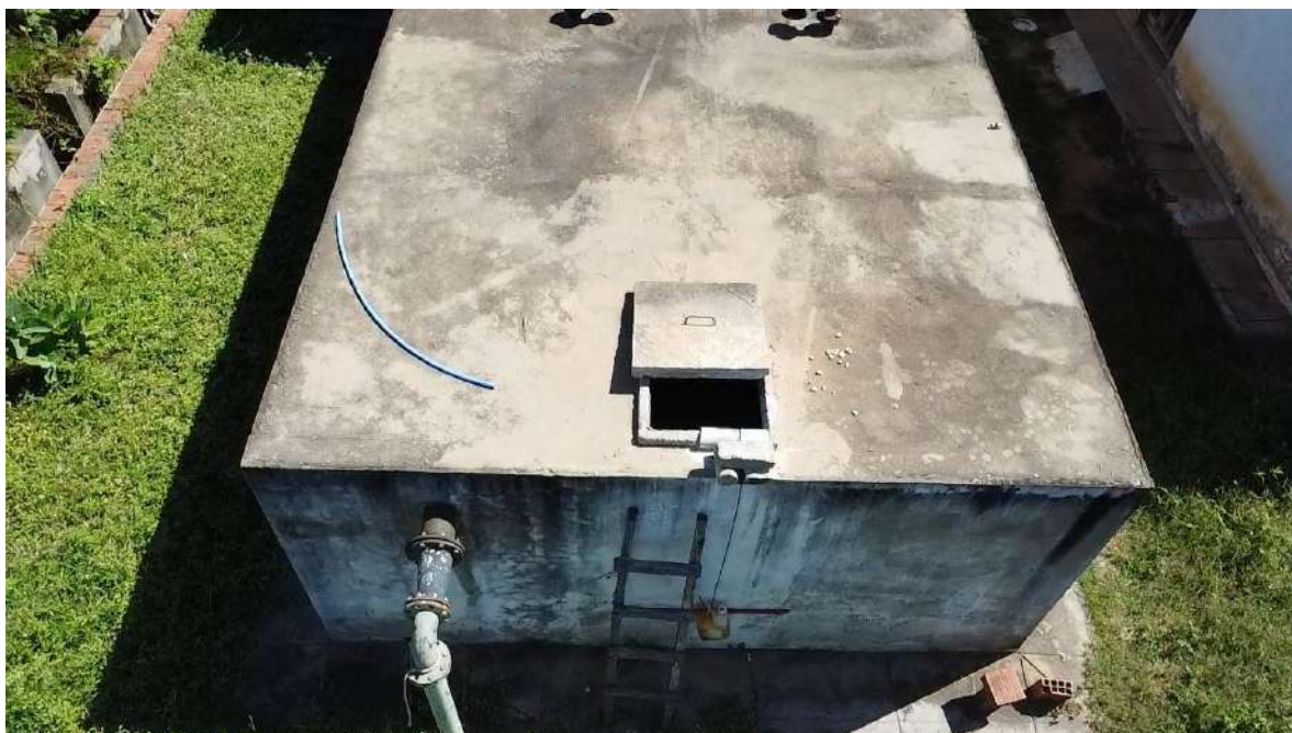
Foto 42 - RAP-06: tampa deslocada, pintura desgastada e escada improvisada, sem fixação.
