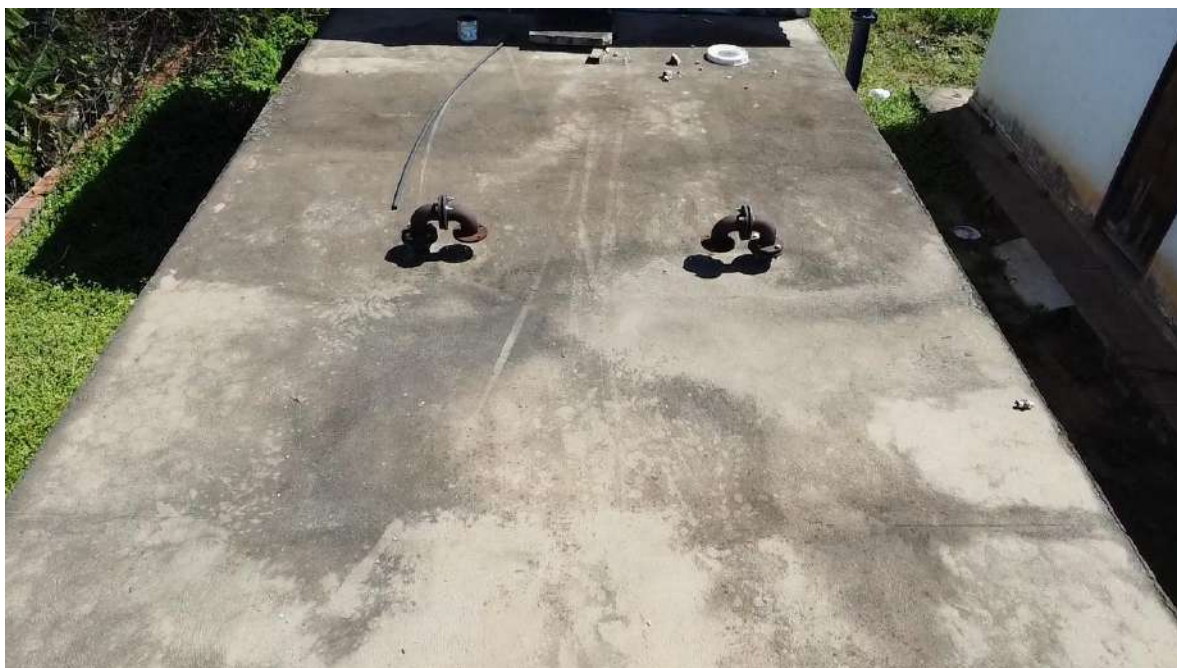
Foto 18 - RAP-06: tubulação de ventilação sem tela de proteção.
