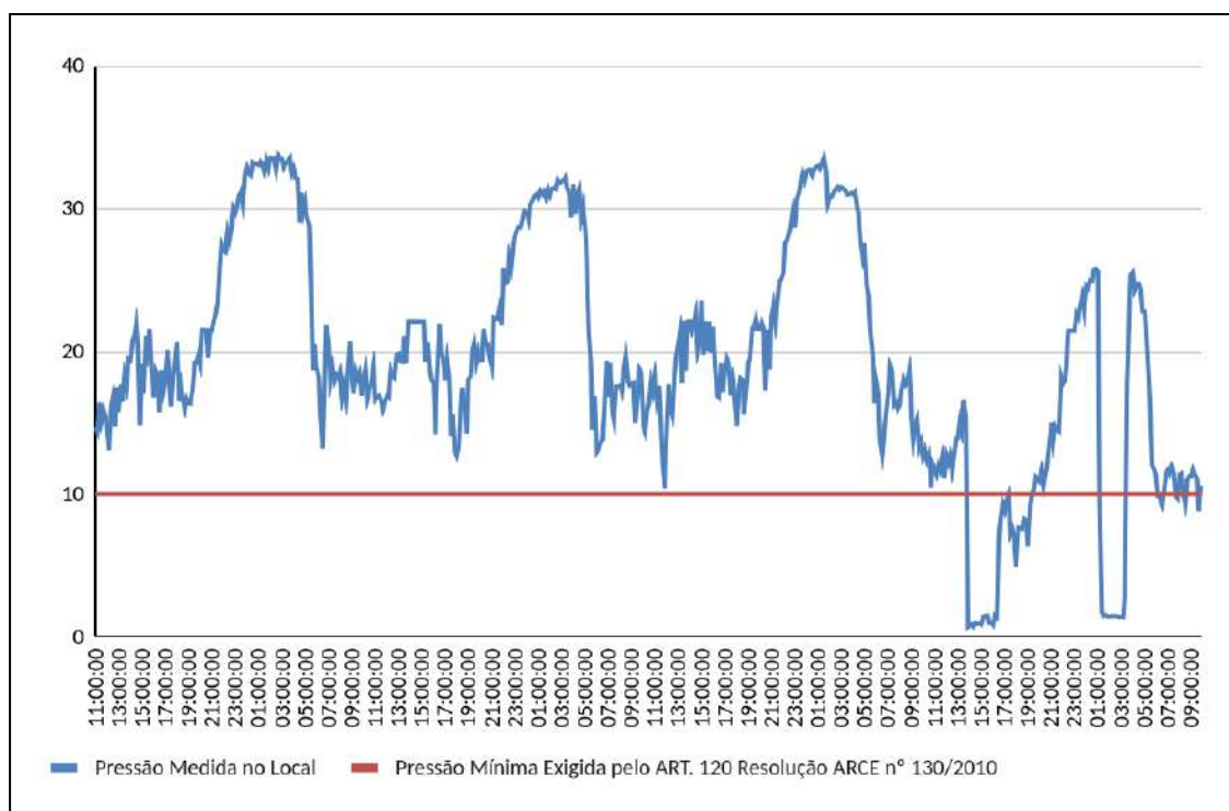
Figura 12 - Monitoramento da pressão no SAA da Localidade de Lagoa de Dentro, de 09/09/2024 a 13/09/2024, no endereço: Rua Pedro Cavalcante, s/n, Lagoa de Dentro.
