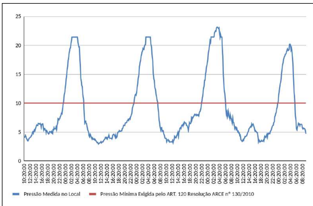
Figura 7 - Monitoramento da pressão no SAA da Sede de Itaitinga, de 04/10/2024 a 08/10/2024, no endereço: Rua Monte Sinai, 223 F.
