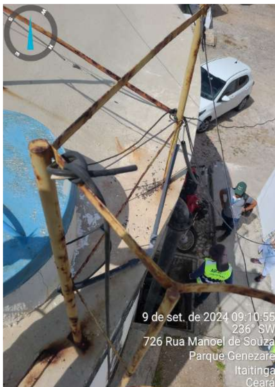
Foto 19 - RAP-01: instalações elétricas inadequadas e escada corroída.
