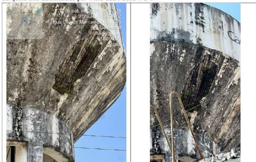
Foto 1 e 2 – Vistas das armaduras expostas do reservatório elevado
