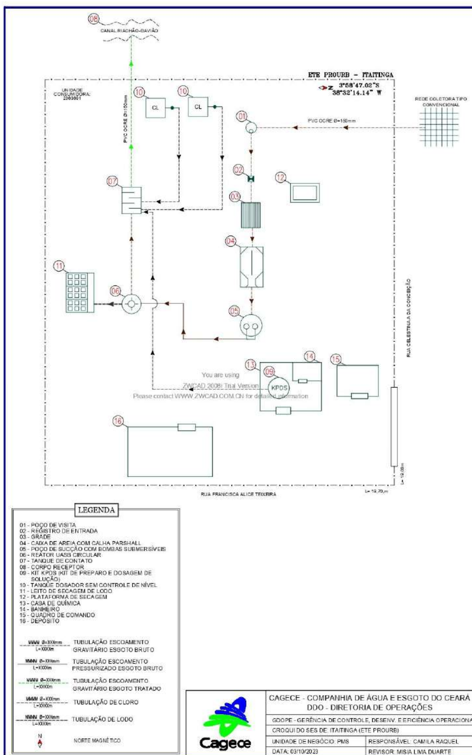
Figura 3 - Croqui do SES - ETE Angorá (Prourb)
