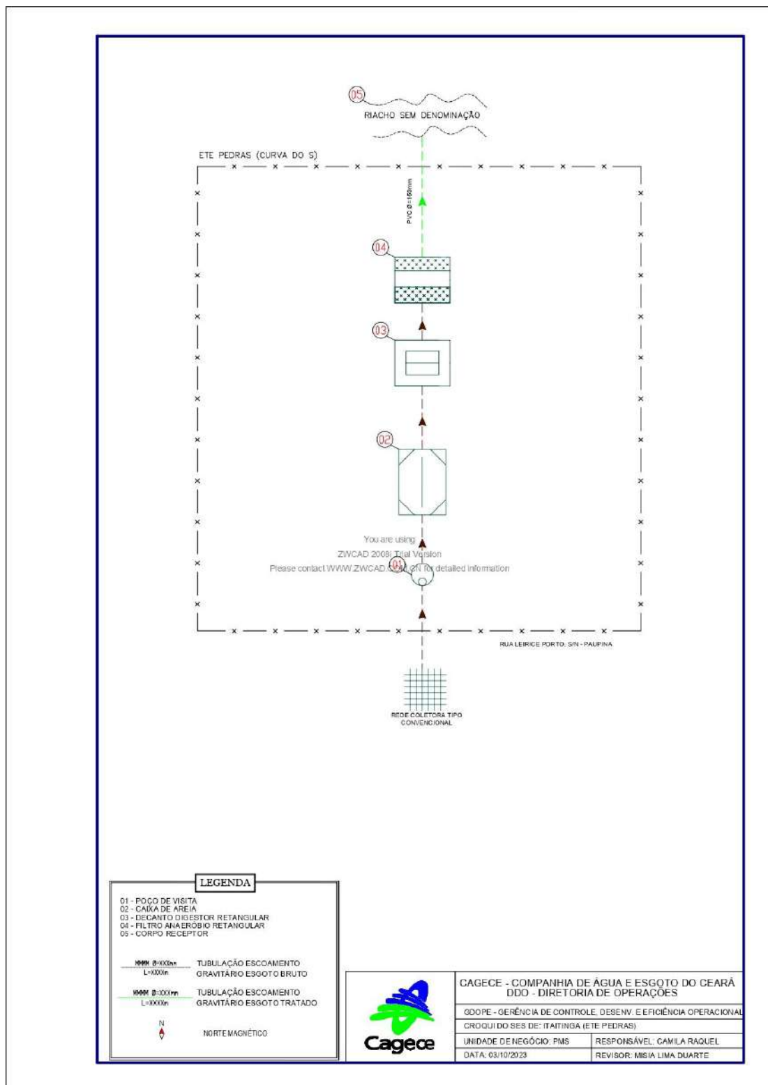
Figura 2 - Croqui do SES - ETE Pedras
