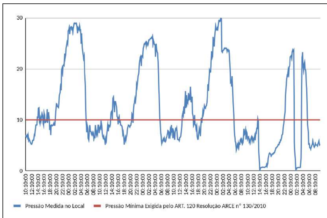
Figura 11 - Monitoramento da pressão no SAA da Localidade de Carapió, de 09/09/2024 a 13/09/2024, no endereço: Rua Antônio Carneiro, 111, Carapió.
