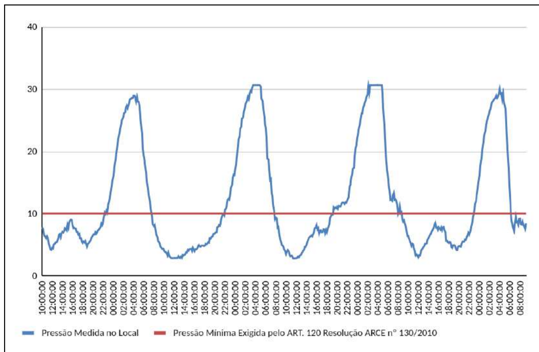
Figura 6 - Monitoramento da pressão no SAA da Sede de Itaitinga, de 04/10/2024 a 08/10/2024, no endereço: Rua Raul Nogueira, 366.
