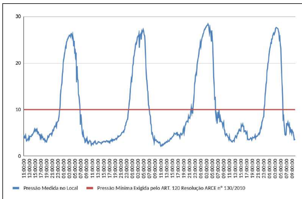
Figura 9 - Monitoramento da pressão no SAA da Sede de Itaitinga, de 04/10/2024 a 08/10/2024, no endereço: Rua José Geraldo, 23.
