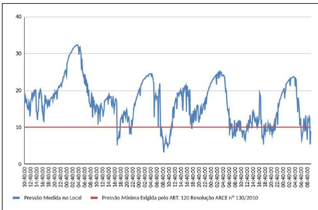
Figura 8 - Monitoramento da pressão no SAA da Sede de Itaitinga, de 04/10/2024 a 08/10/2024, no endereço: Rua Santa Luzia, 411.
