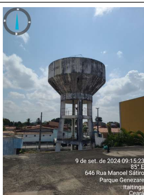
Foto 2 - REL-01: escada e guarda-corpo corroídos, pintura deteriorada e estrutura em concreto armado com aço exposto.
