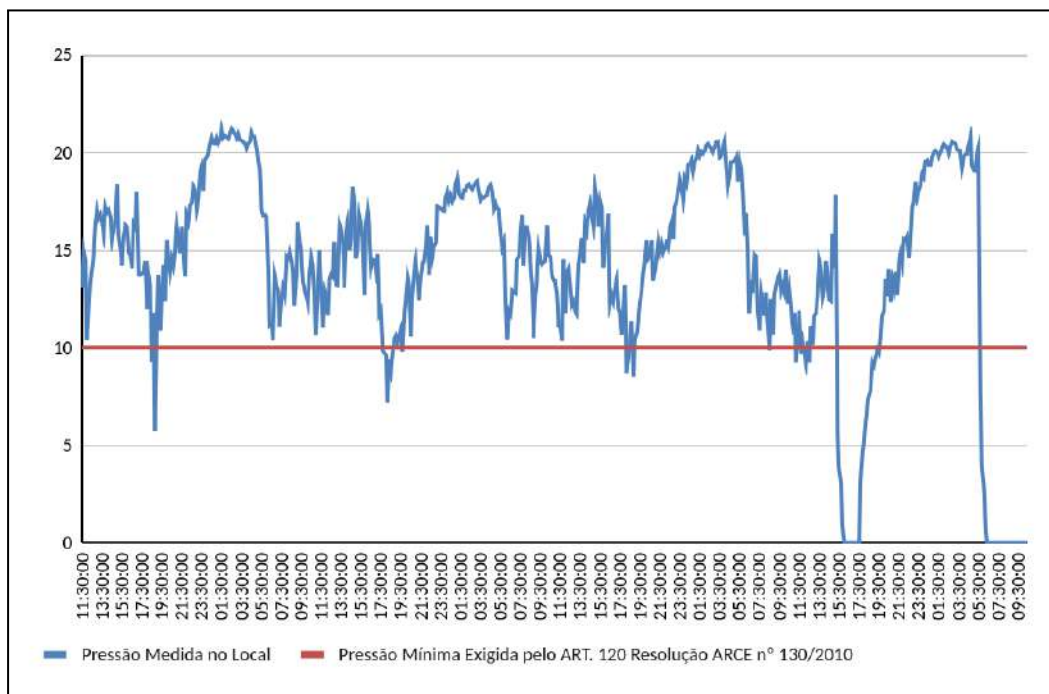
Figura 10 - Monitoramento da pressão no SAA da Localidade de Riachão, de 09/09/2024 a 13/09/2024, no endereço: Rua Paulo Tavares da Rocha, 365, Genezaré, Riachão.
