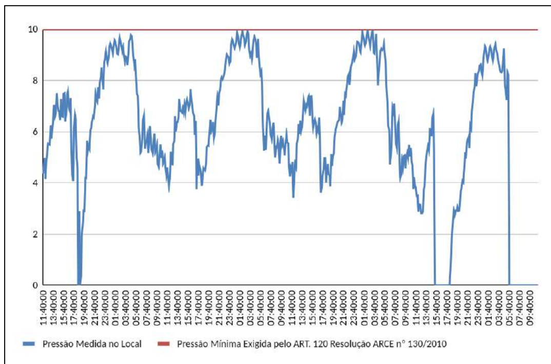
Figura 5 - Monitoramento da pressão no SAA da Sede de Itaitinga, de 09/09/2024 a 13/09/2024, no endereço: Rua Lauro Ferreira Viana, 228, Centro.
