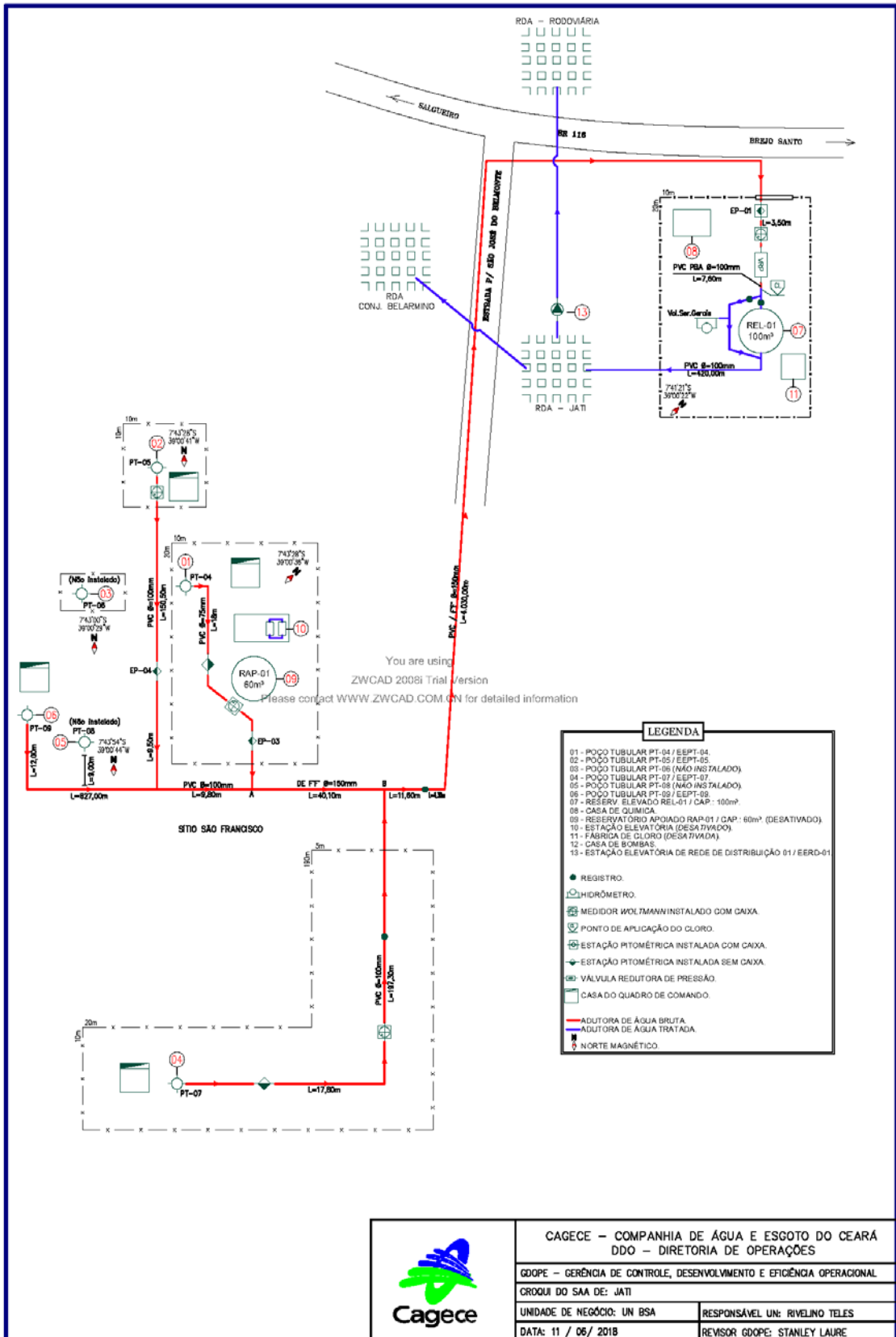
Figura 4.4 - Croqui do SAA da zona URBANA do Distrito Sede de Jati, 2018
