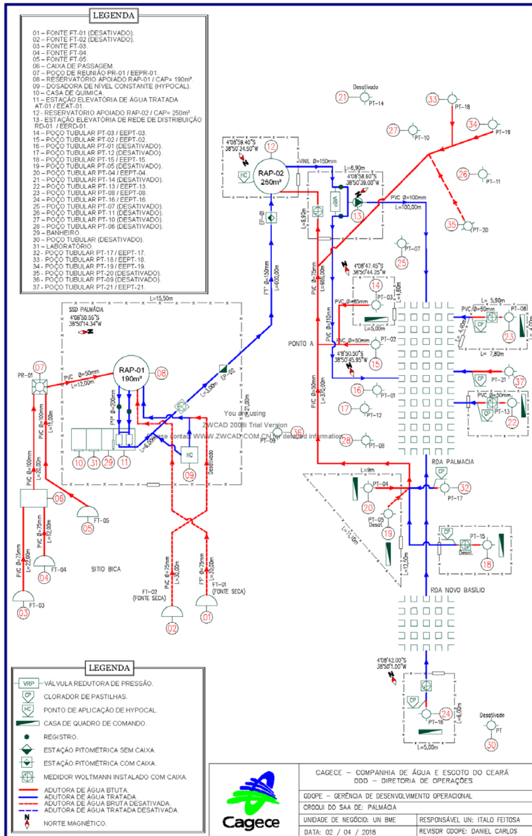
Figura 4.2 - Croqui do SAA da zona URBANA do Distrito Sede de Palmácia, 2018
