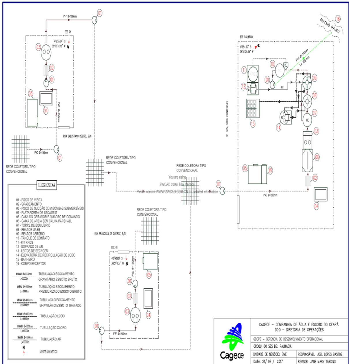
Figura 4.3 - Croqui do SES da zona urbana de Palmácia
